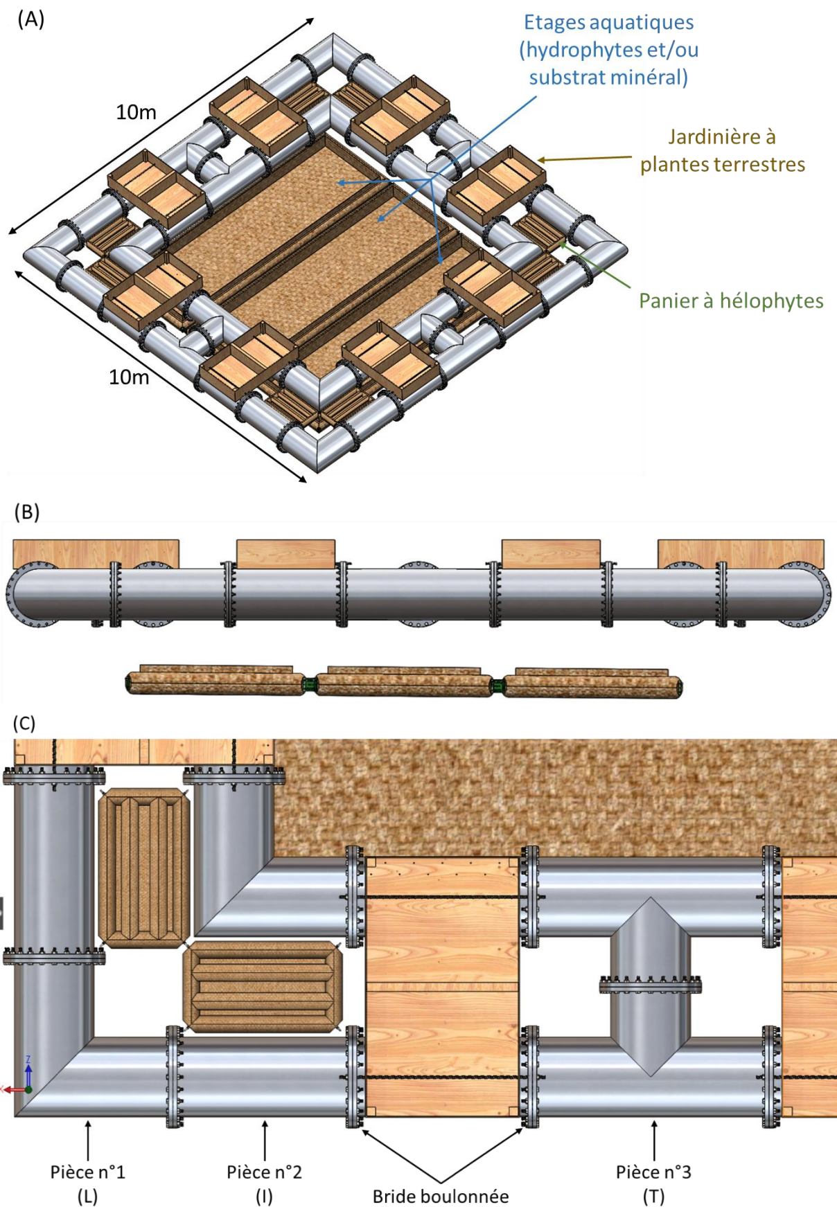
Figure 9 : Esquisse 3D de la conception finale des FLOLIZs. (A) Vue \frac{3}{4} avec annotations ; (B) Vue de profil ; (C) Zoom sur les différentes pièces. ©ECOCEAN
